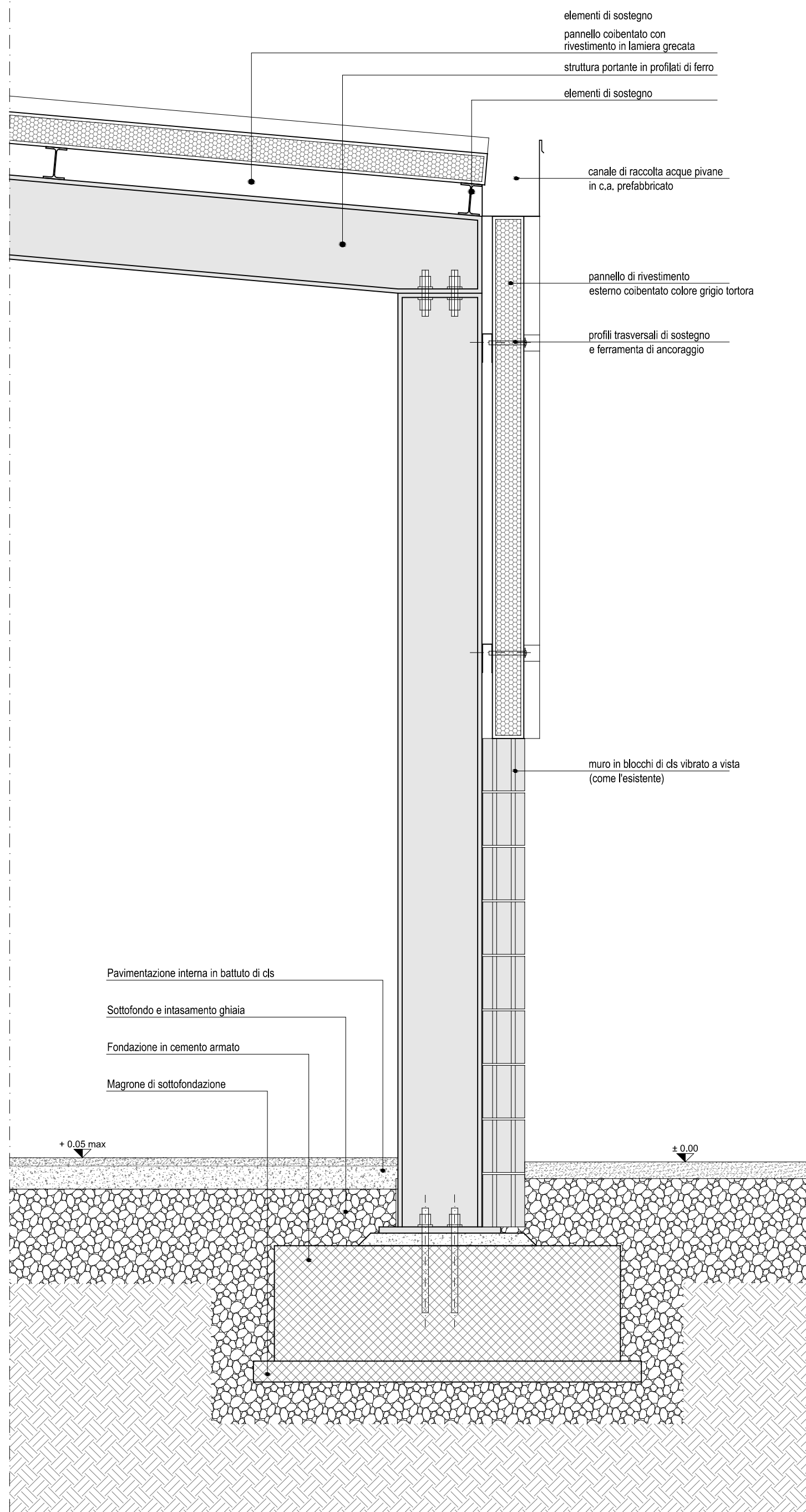
Particolare costruttivo sc. 1:20
